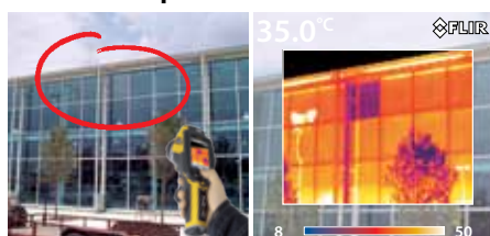
L'inspection thermographique révèle une fenêtre incorrectement installée.
