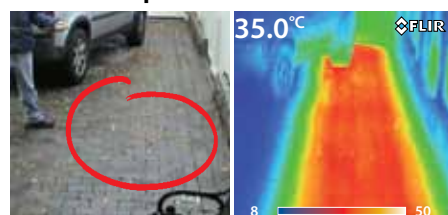
Seule une partie de ce dallage chauffant fonctionne.
