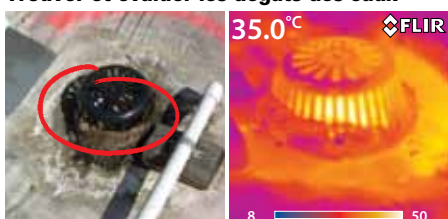
L'image thermique montre une fuite d'eau dans le toit.
